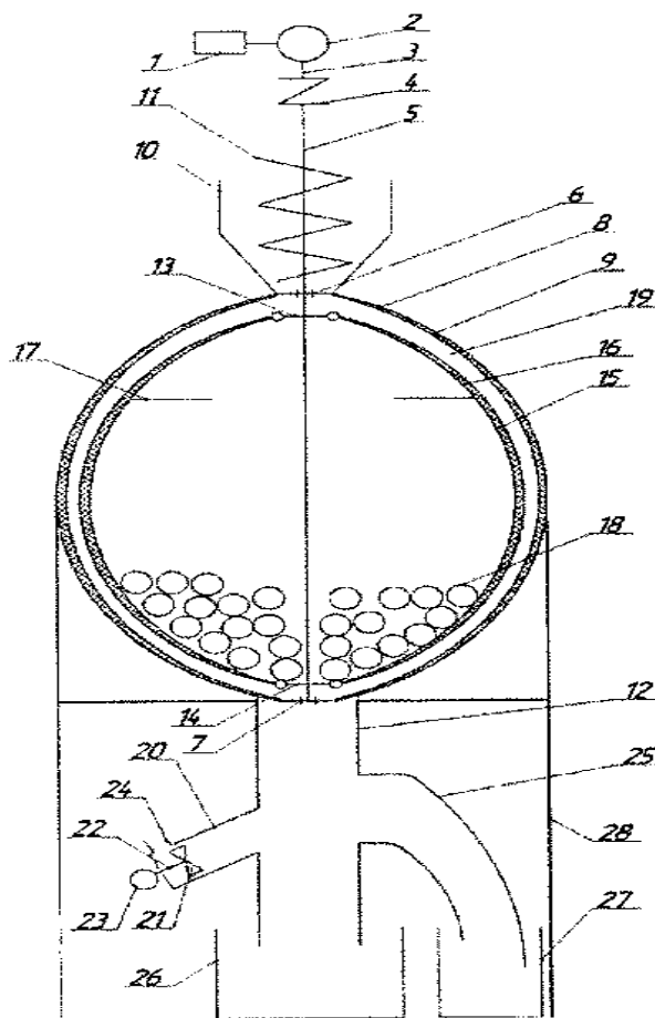
Рисунок 3 – Общий вид шелушителя
