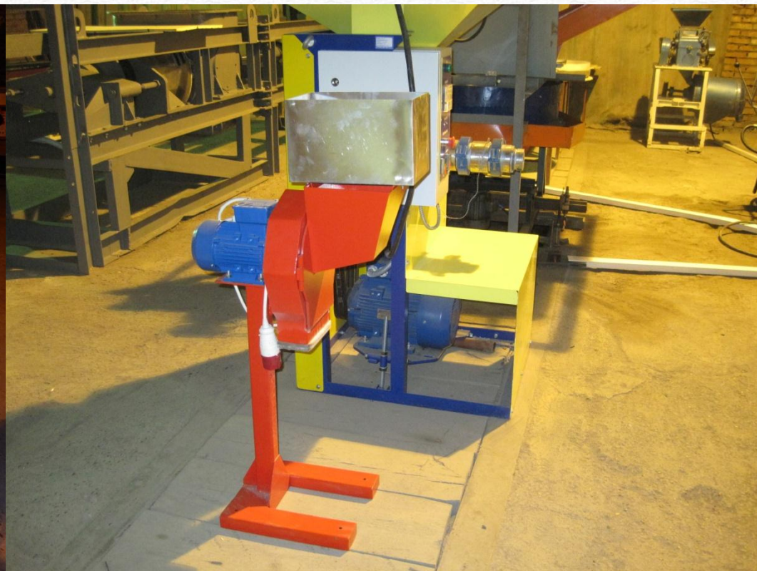
Дробилка молотковая
