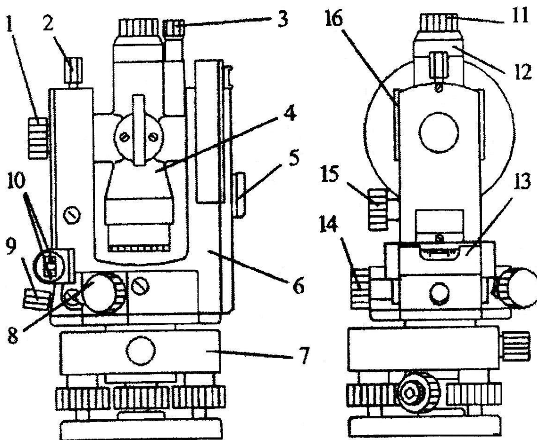
Рисунок 4 – Устройство теодолита 4Т30П:
