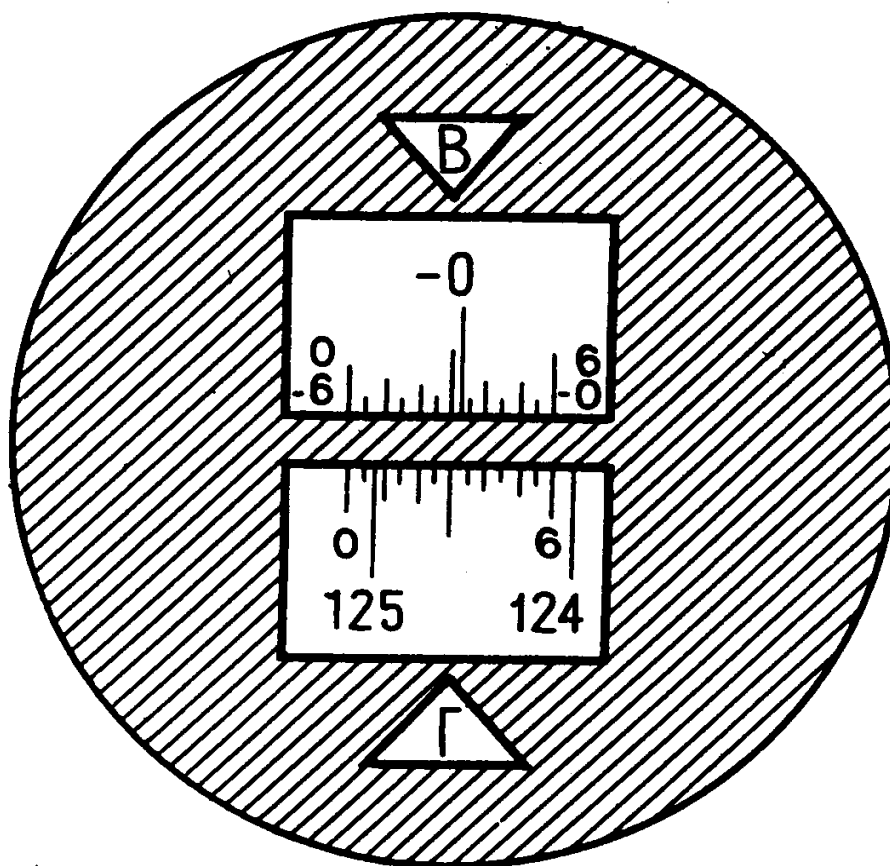
Рисунок 5 – Поле зрения микроскопа теодолита 4Т30П с ценой деления шкалы 5'
