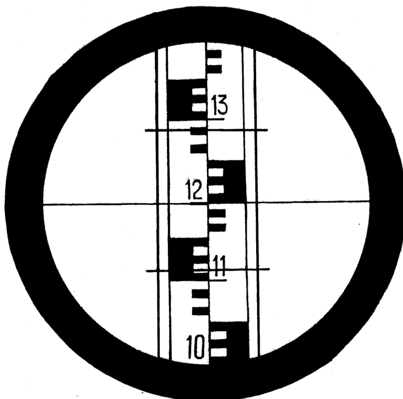
Рисунок 7 – Поле зрения зрительной трубы теодолита 4Т30П
