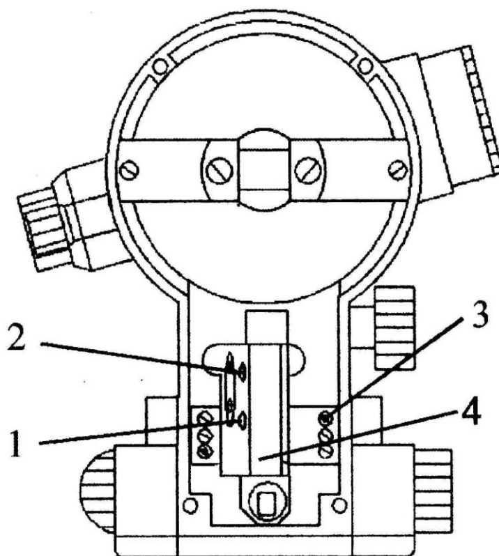
Рисунок 9 – Теодолит 4Т30П без боковой крышки 1, 2 – винты крепления линз горизонтального круга; 3 – винт крепления кронштейна; 4 – кронштейн
