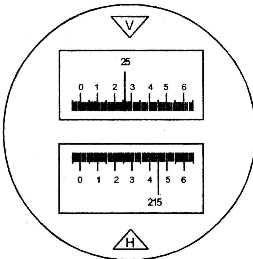
Рисунок 6 – Поле зрения микроскопа теодолита 4Т30П с ценой деления шкалы 1'
