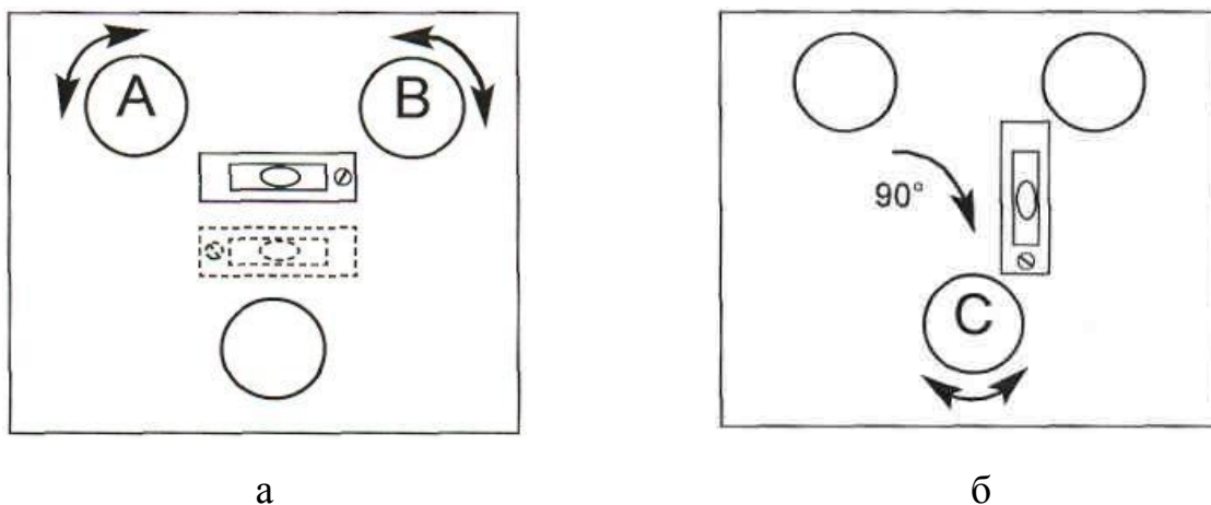
Рисунок 8 – Точное горизонтирование по цилиндрическому уровню
