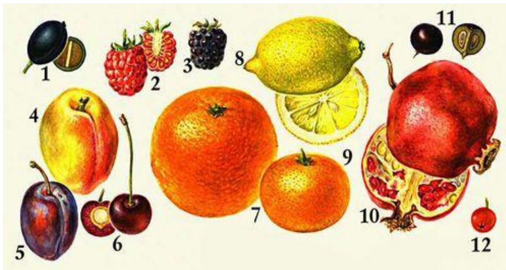
Рисунок 15 – Апокарпные плоды:
