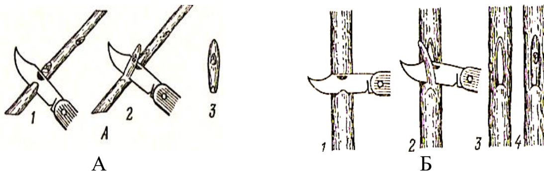
Рисунок 20 – Окулировка в приклад:
