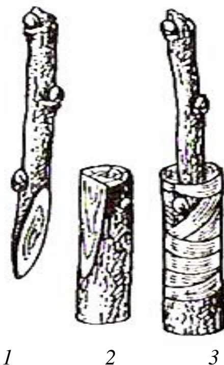
Рисунок 24 – Простая копулировка:
