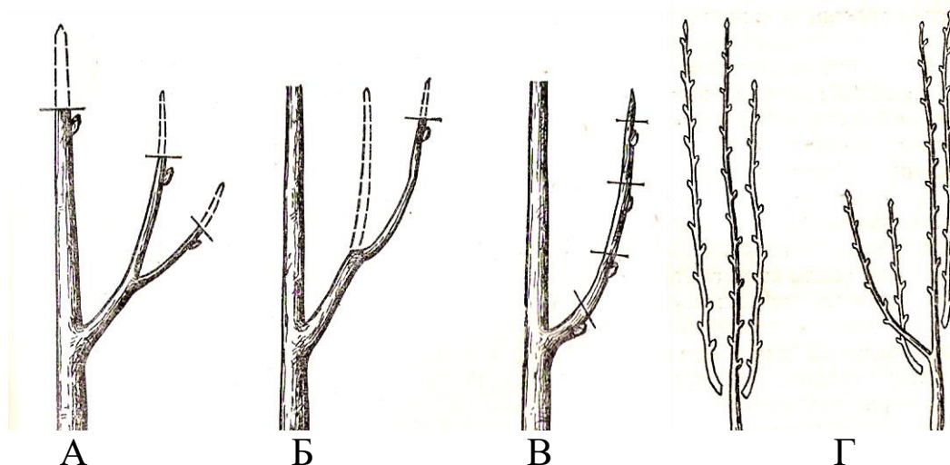
Рисунок 30 – приемы обрезки:
