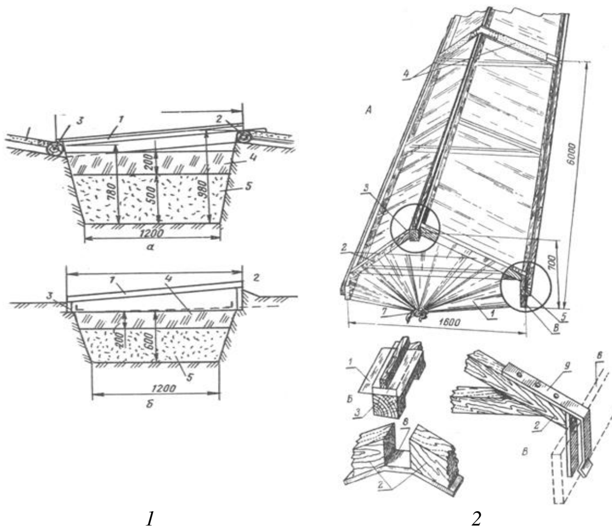
Рисунок 8 – Характеристика парников:
