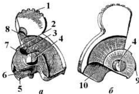
Рис. 9.28. Курок: а – левая сторона; б – правая сторона; 1 – головка с насечкой; 2 – выступ; 3 – выем; 4 – цапфы; 5 – зуб самовзвода; 6 – углубление; 7 – предохранительный взвод; 8 – вырез; 9 – боевой взвод; 10 – кольцевой выем
