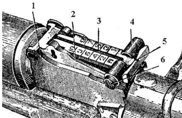
Рис. 9.9. Прицел:
