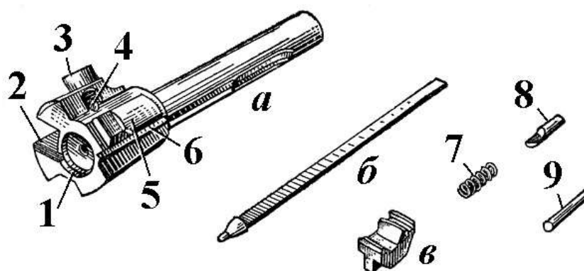
Рис. 9.11. Затвор:
