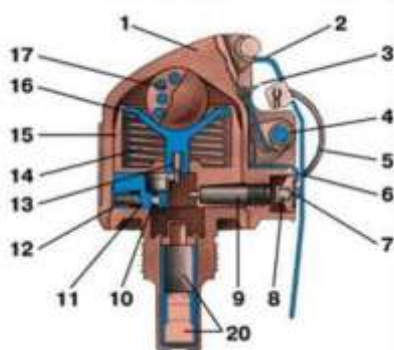
Рис. 9.62. Устройство УДЗ:
