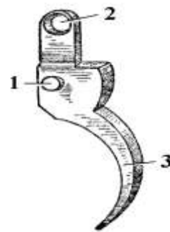
Рис. 9.27. Спускной крючок: 1 – цапфа; 2 – отверстие для соединения со спусковой тягой; 3 – хвост
