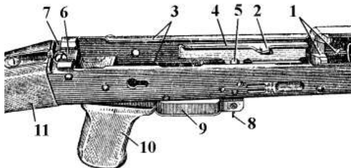
Рис. 9.8. Ствольная коробка:
