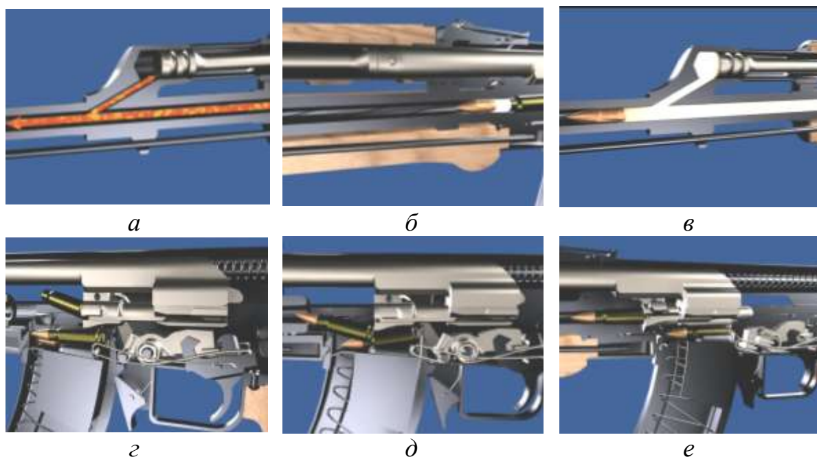
Рис. 9.3. Цикл работы автомата Калашникова
