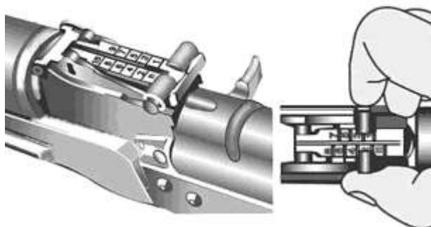
Рис. 9.41. Установка прицела
