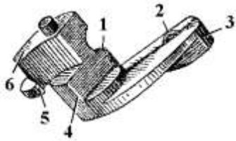
Рис. 9.21. Предохранитель: 1 – уступ; 2 – фиксатор; 3 – флажок предохранителя; 4 – ребро; 5 – зацеп; 6 – выступ
