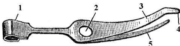
Рис. 9.30. Боевая пружина: 1 – защелка; 2 – отверстие; 3 – широкое перо; 4 – отбойный конец; 5 – узкое перо
