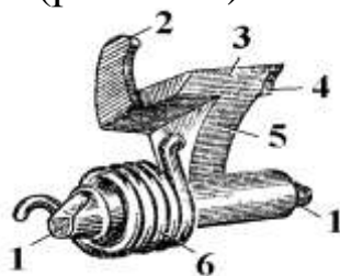
Рис. 9.29. Шептало: 1 – цапфы шептала; 2 – зуб; 3 – носик шептала; 4 – выступ; 5 – стойка шептала; 6 – пружина шептала
