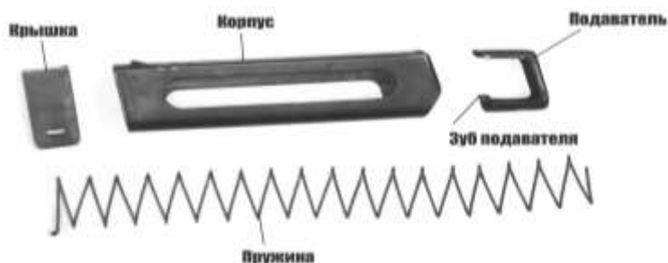
Рис. 9.32. Магазин
