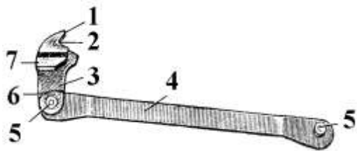
Рис. 9.26. Спускная тяга с рычагом взвода: 1 – разобцающий выступ рычага взвода; 2 – вырез; 3 – рычаг взвода; 4 – спусковая тяга; 5 – цапфы спусковой тяги; 6 – пяточка рычага взвода; 7 – выступ самовзвода
